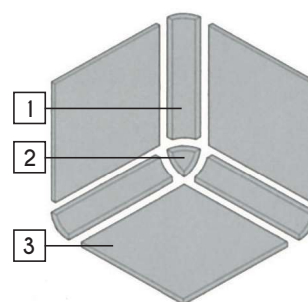
1. Escocia 5x20 2. Ángulo Escocia 5x5 3. Azulejo 20x20
