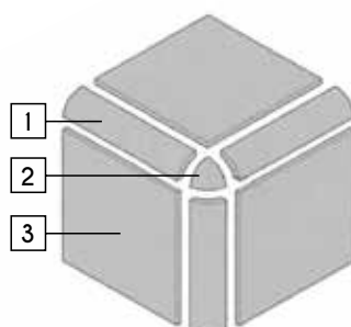
1. Cubrecanto 5x20 2. Ángulo Cubrecanto 5x5 3. Azulejo 20x20
